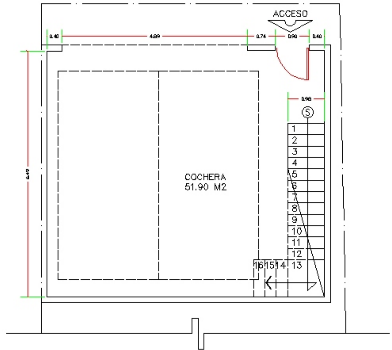
2 PLANTA ARQUITECTONICA ESC: 1.50 COCHERA 51.90 M2
