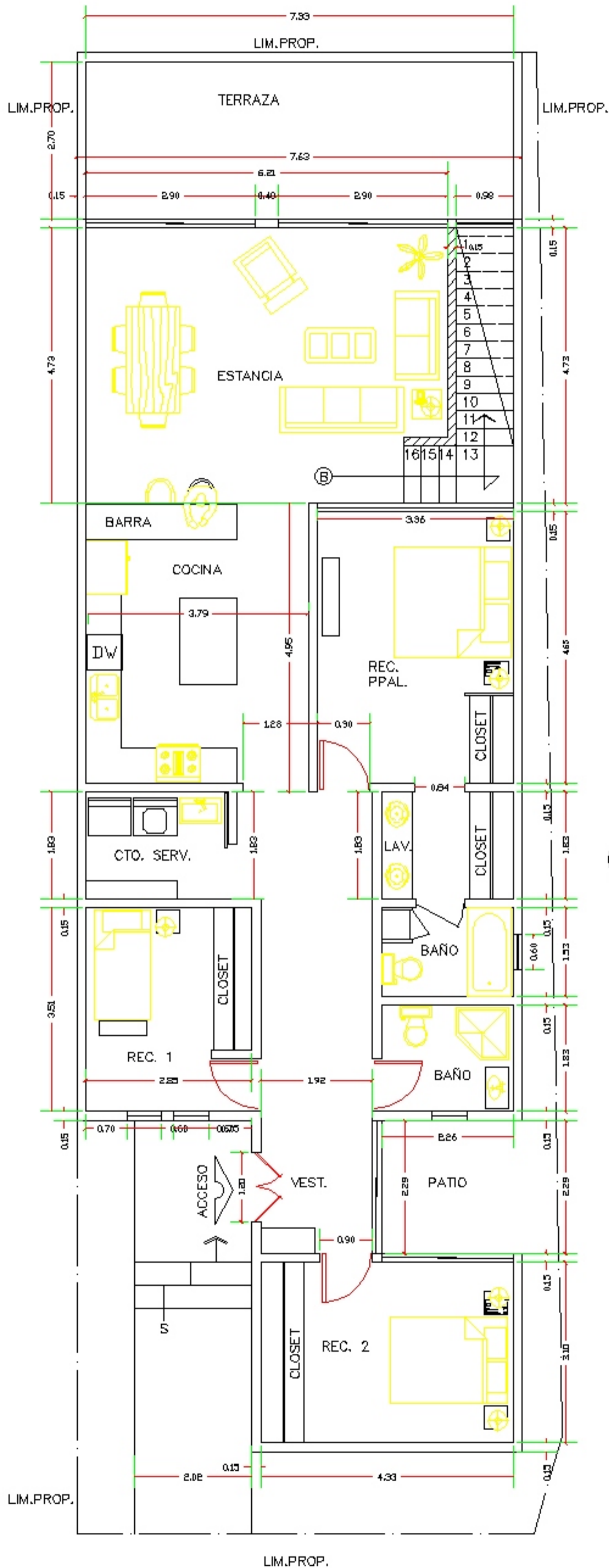
1 PLANTA ARQUITECTONICA ESC: 1.50 PLANTA BAJA. SUP: 138.85 M2 TERRAZA: 21.75 M2
